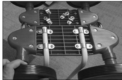
6. Przymocuj pozostałe 2 łączniki
